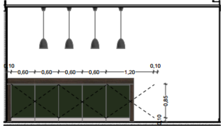
AI-03 03 ELEVACIÓN SECTOR BAR 1:50
